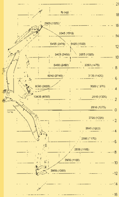
BRAZO CON AGUILÓN EXTENSIBLE HED, CORTO RETRAIDO Y CUCHARA HD 610 mm (156 kg) / Cuchara de Cargadora 6 x 1
