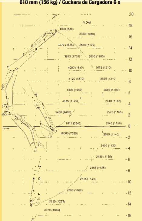
BRAZO CON AGUILÓN EXTENSIBLE HED LARGO EXTENDIDO CON CUCHARA HD 610 mm (156 kg) / Cuchara de Cargadora 6 x 1
