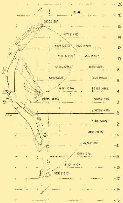
BRAZO CON AGUILÓN ESTÁNDAR Y CUCHARA HD 610 mm (156 kg) / Cuchara de Cargadora 6 x 1
