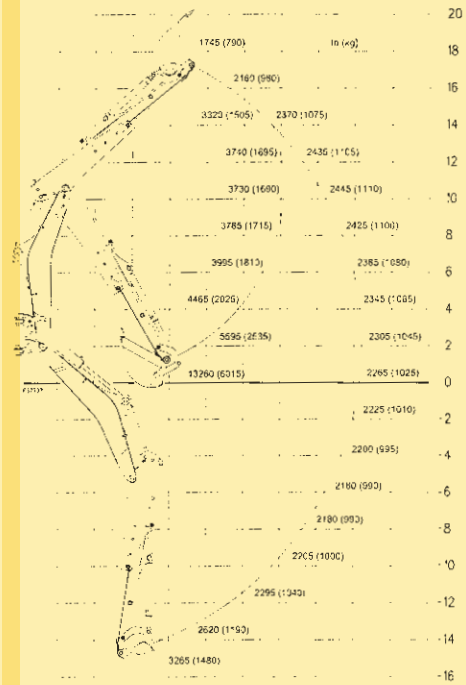
BRAZO CON AGUILÓN EXTENSIBLE HED, CORTO EXTENDIDO Y CUCHARA HD 610 mm (156 kg) / Cuchara de Cargadora 6 x 1
